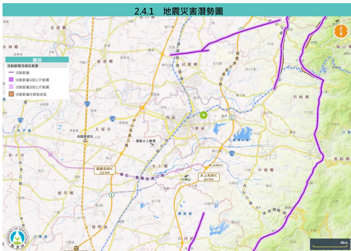
圖 2.4.1 地震災害潛勢圖 (瀏覽日期：110 年 04 月 06 日)
